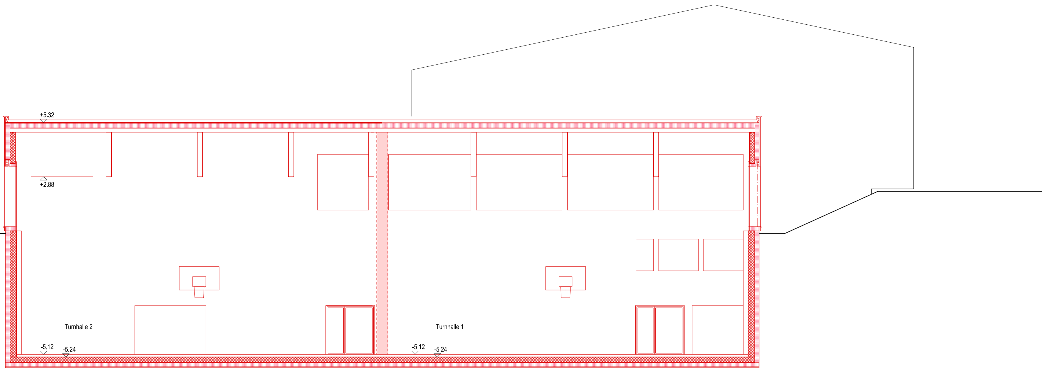
Querschnitt A - A
